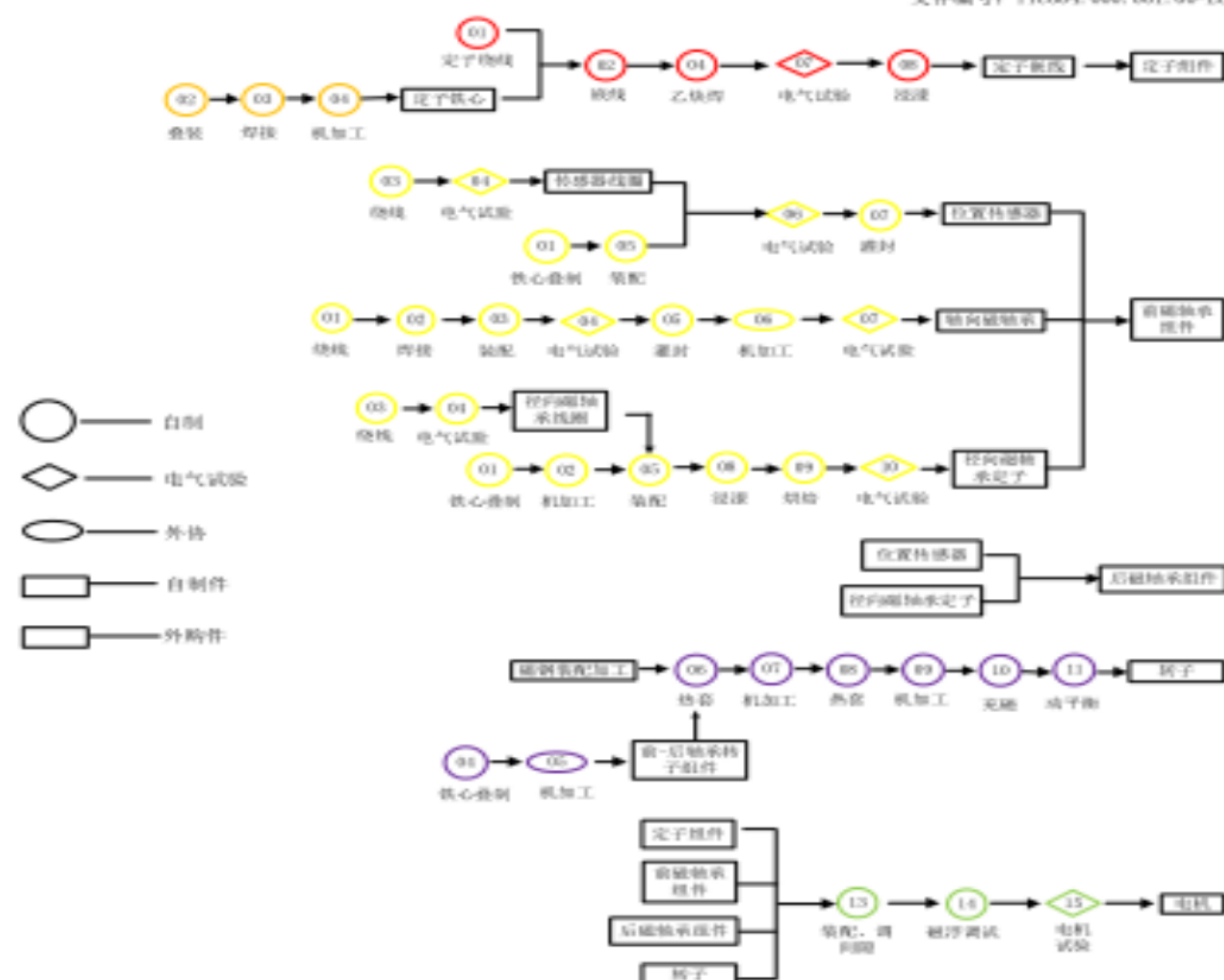
XV150B01同步永磁高速电机工艺流程图
