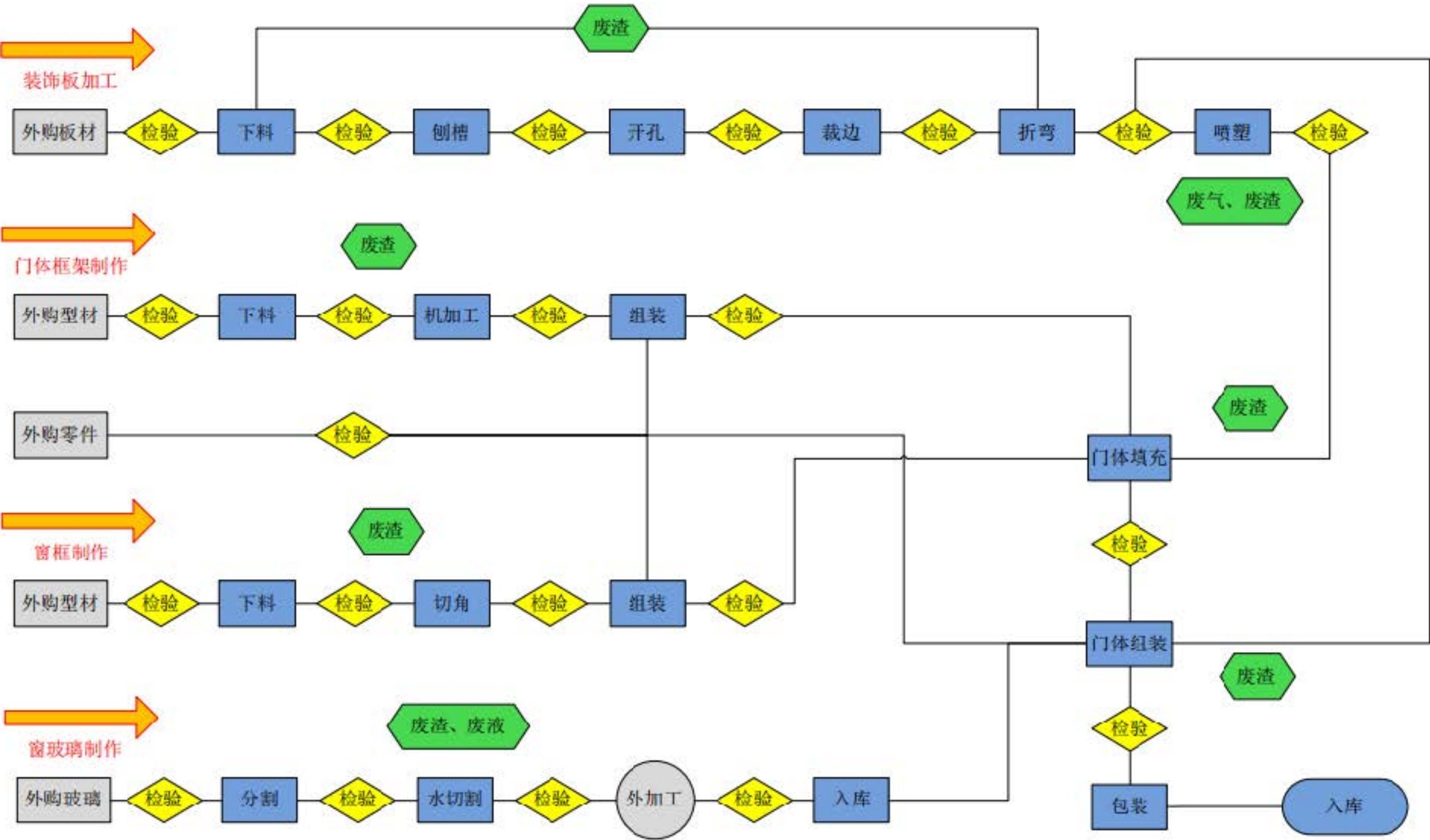
门体制作工艺流程图
