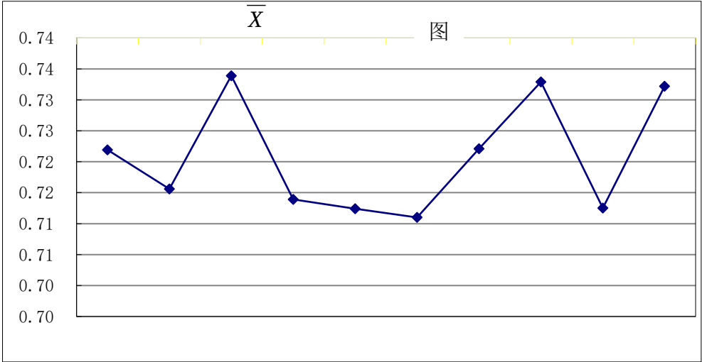
\bar{x} - s图
