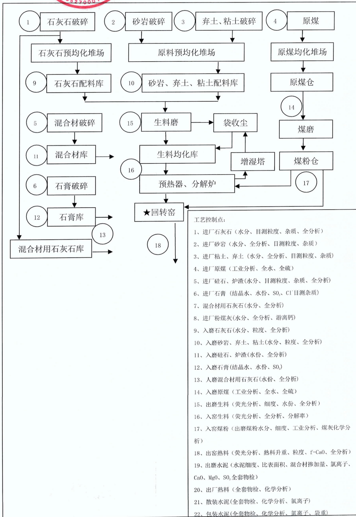
附录 3：工艺流程图
