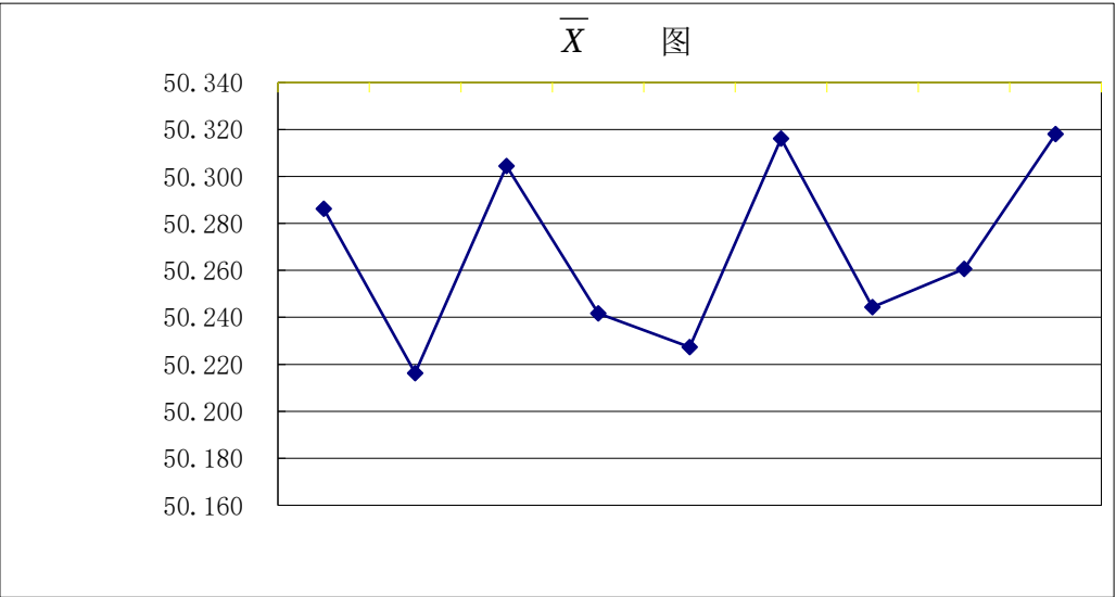
\bar{X} - s图
