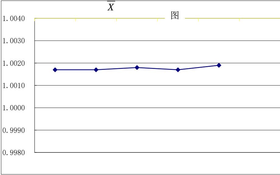
\bar{X} - s 图
