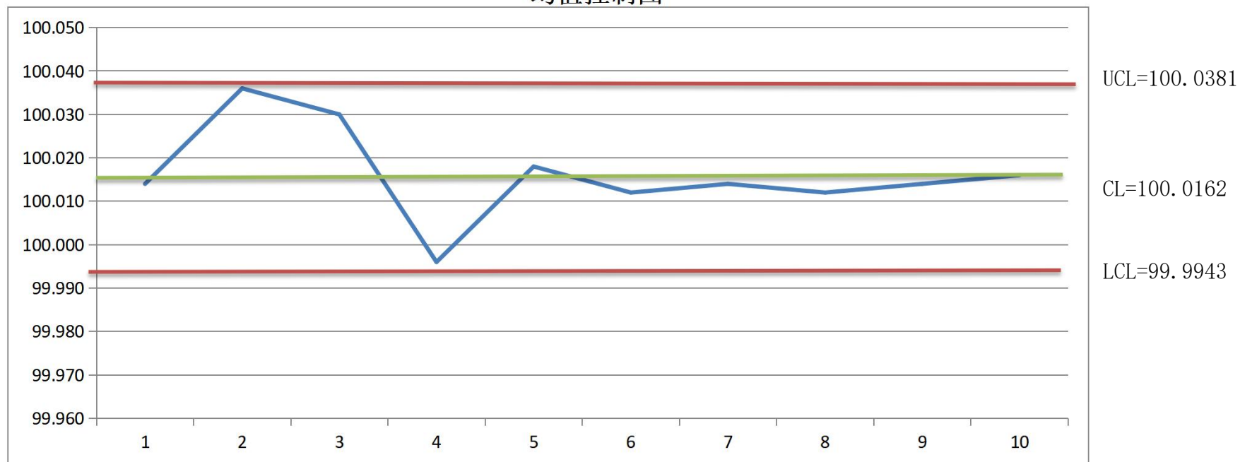
均值控制图
