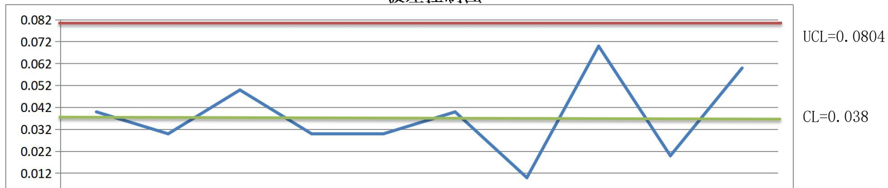
极差控制图
