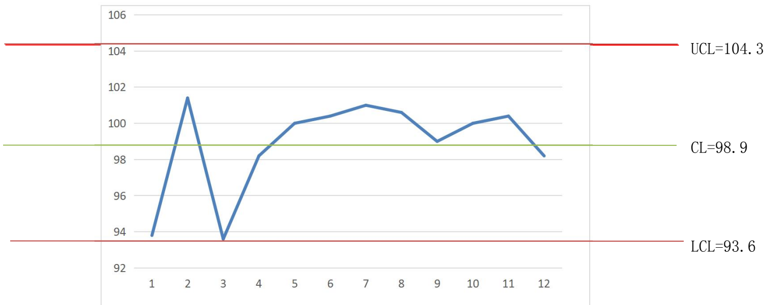
均值控制图
