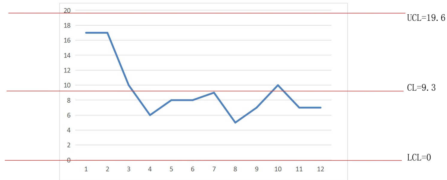
极差控制图
