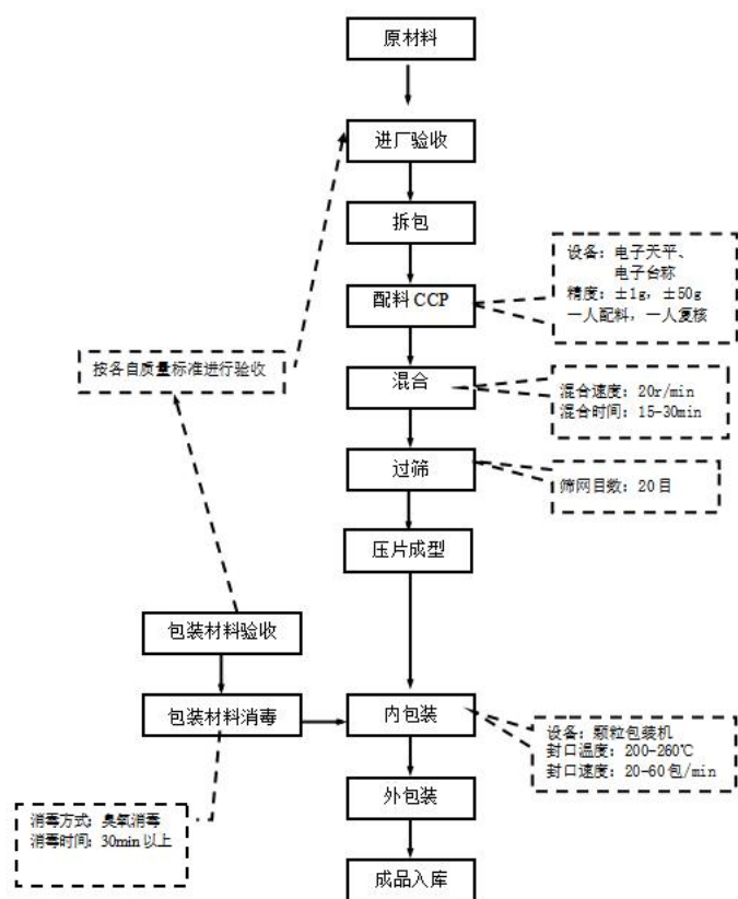
糖果（压片糖果）生产工艺流程图
