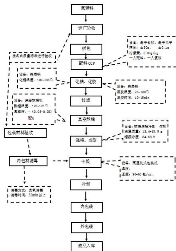
(2)糖果（凝胶糖果）生产工艺流程图
