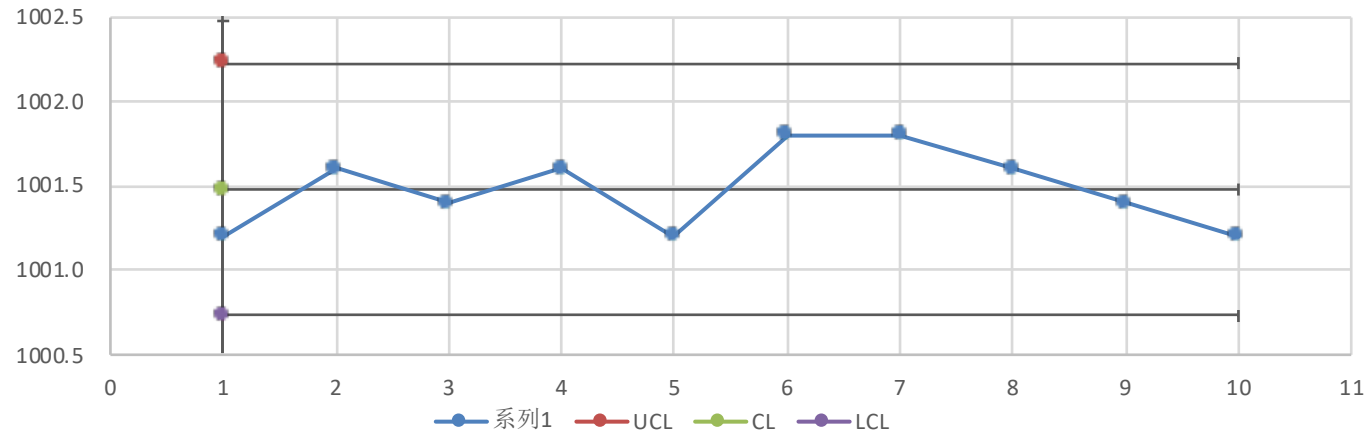
极差控制图
