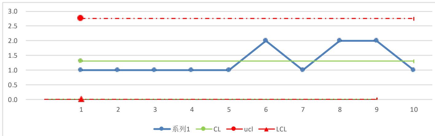
极差控制图
