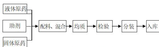
悬浮乳剂生产工艺流程图
