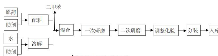
悬浮剂生产工艺流程图
