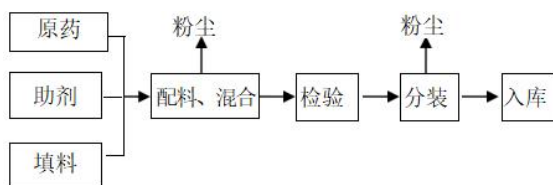
粒剂生产工艺流程图
