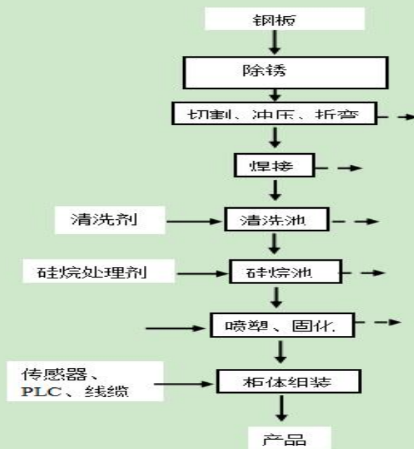
撬装电控一体化产品工艺流程图
