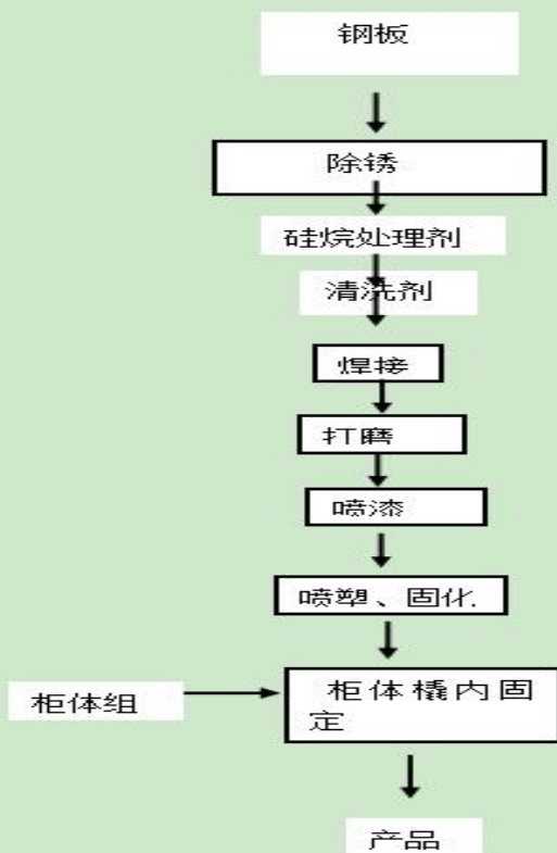
撬装电控一体化产品工艺流程图
