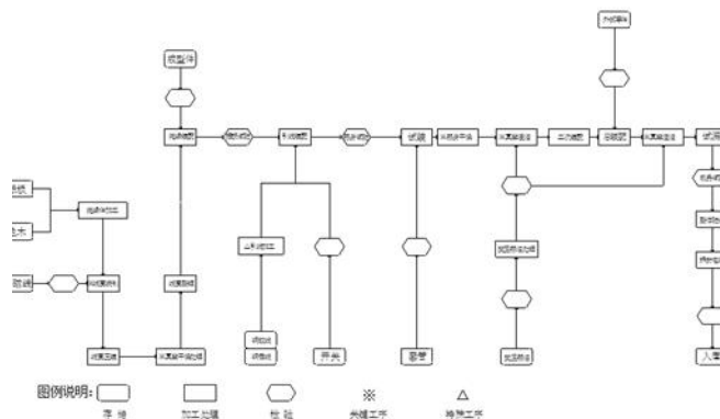
变压器工艺流程图
