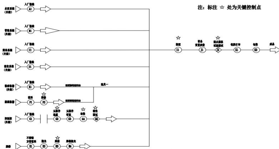
一体化预制泵站工艺流程图：
