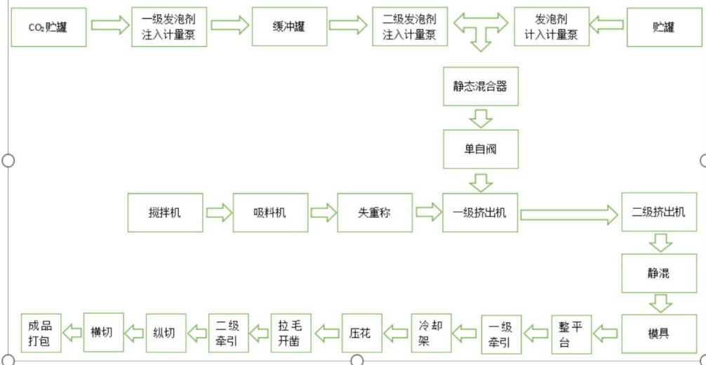
XPS 挤塑保温板生产流程图
