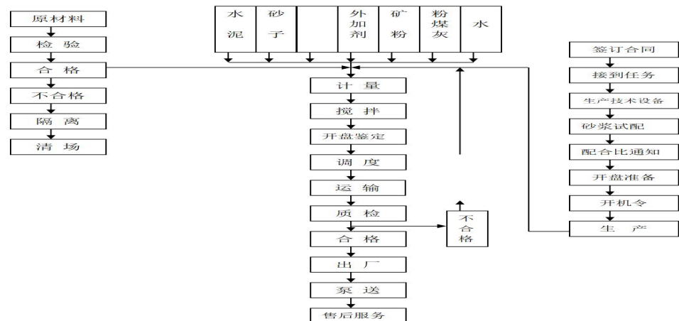
预拌干粉砂浆生产工艺流程
