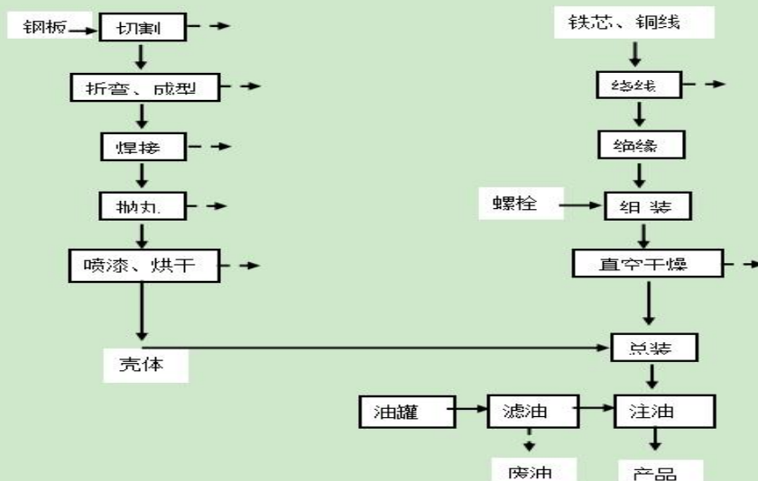
变压器工艺流程图
