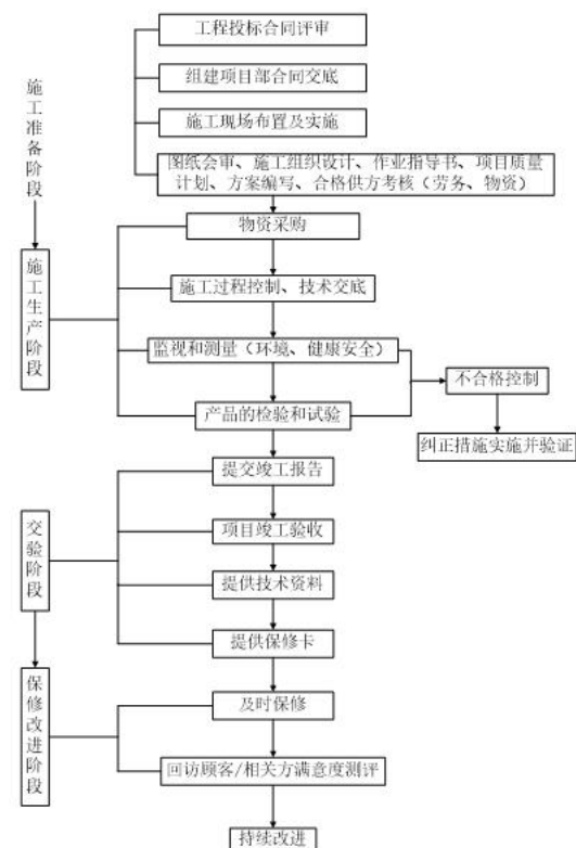
附录 D 施工工艺流程
