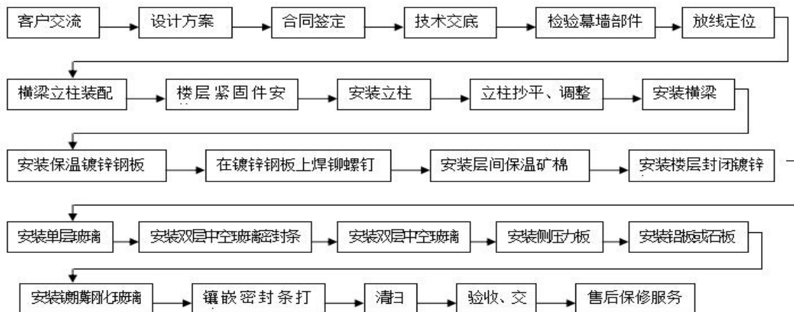
幕墙装饰工程施工工艺流程图
