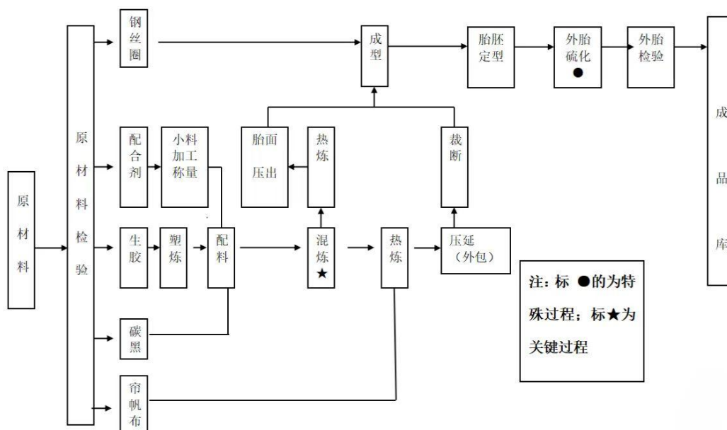
外胎工艺流程图
