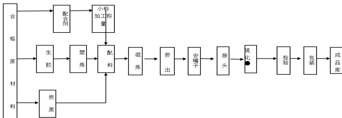
内胎工艺流程图
