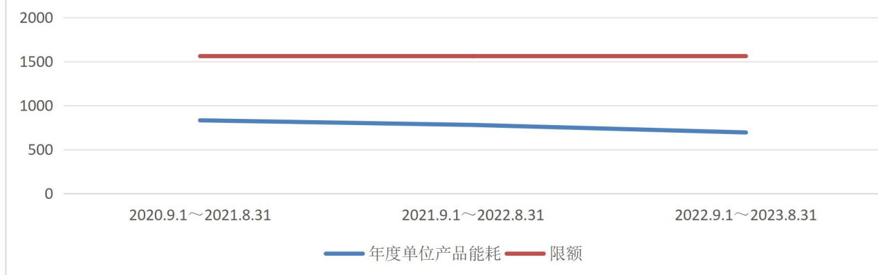
单位产品能耗走势图
