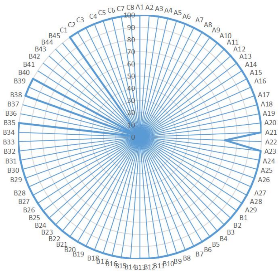
分项得分%
