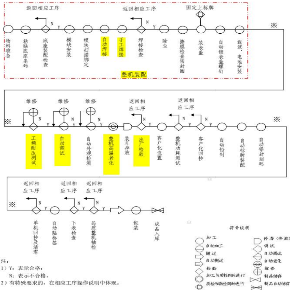
整机受控工艺流程图 (有铅)
