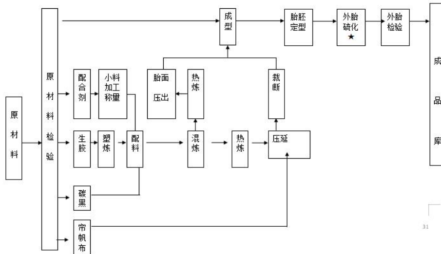
外胎工艺流程图
