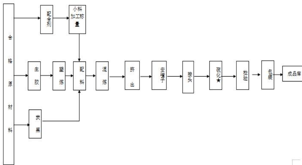
内胎工艺流程图
