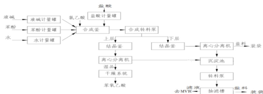
苯氧乙酸流程简图
