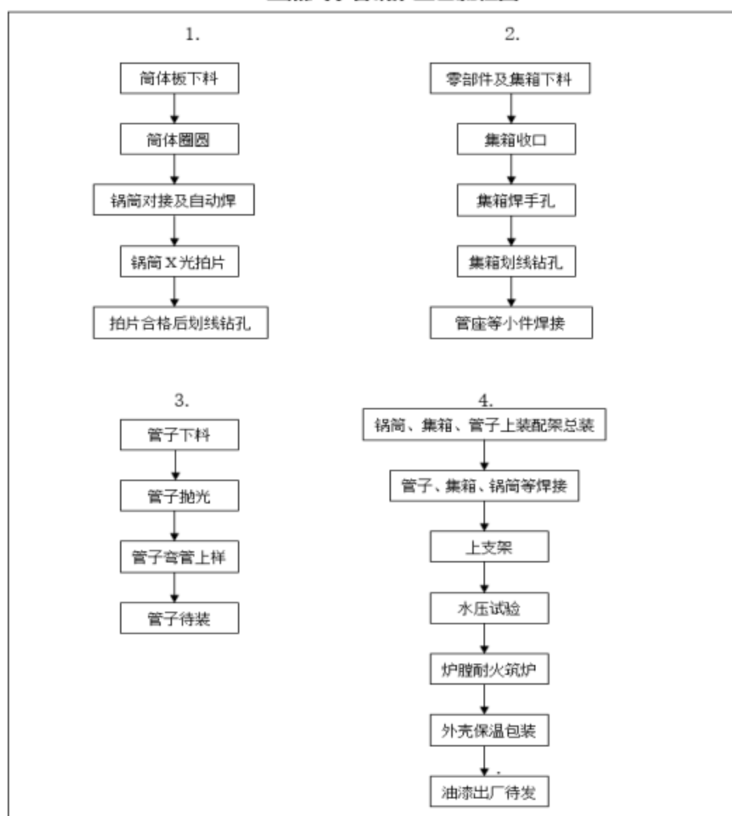
SZL 型蒸汽水管锅炉工艺流程图
