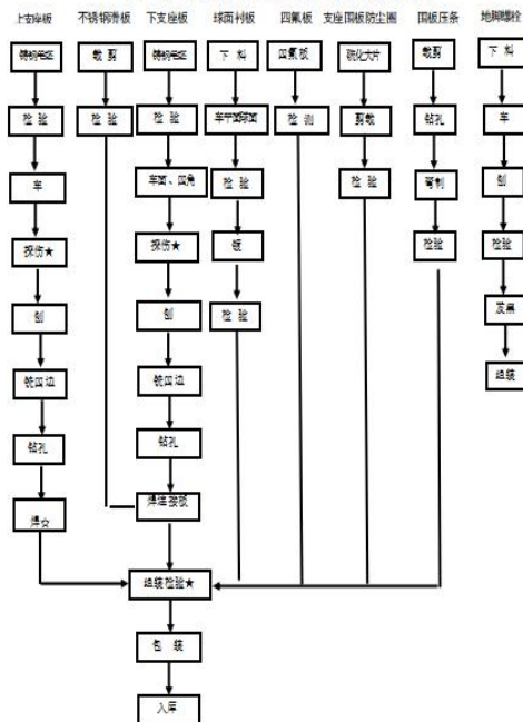
(三)、球型支座生产工艺流程图
