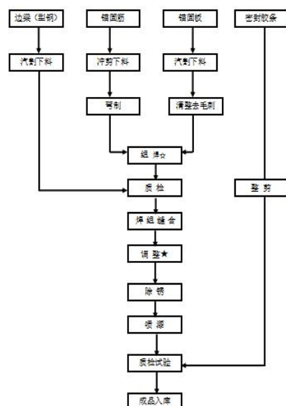
(四)、伸缩缝生产工艺流程图
