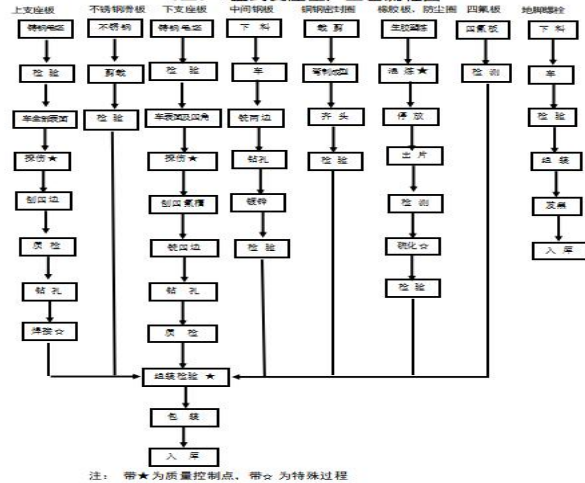
(二)、盆式支座生产工艺流程图
