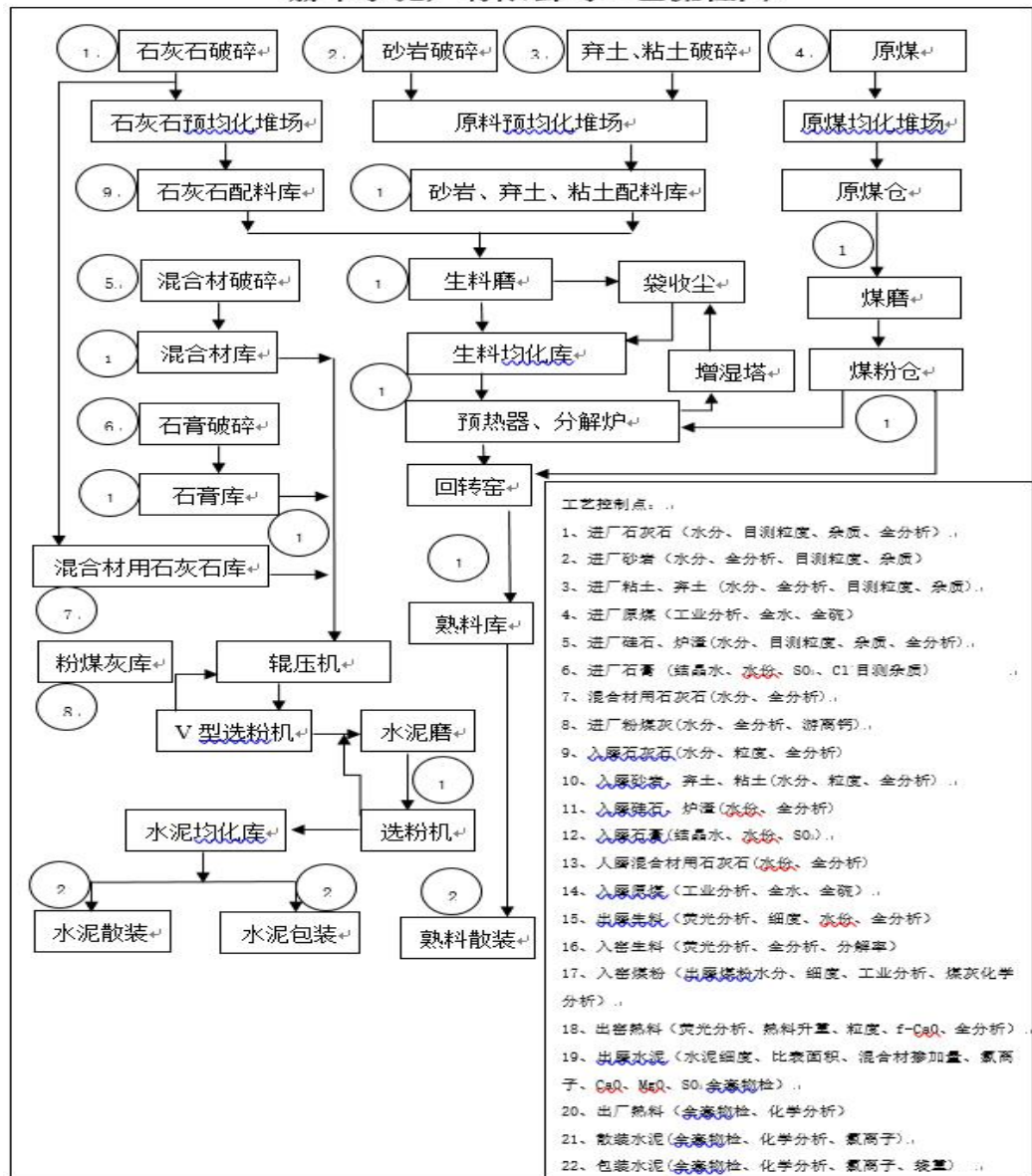
赫章水泥厂有限公司工艺流程图
