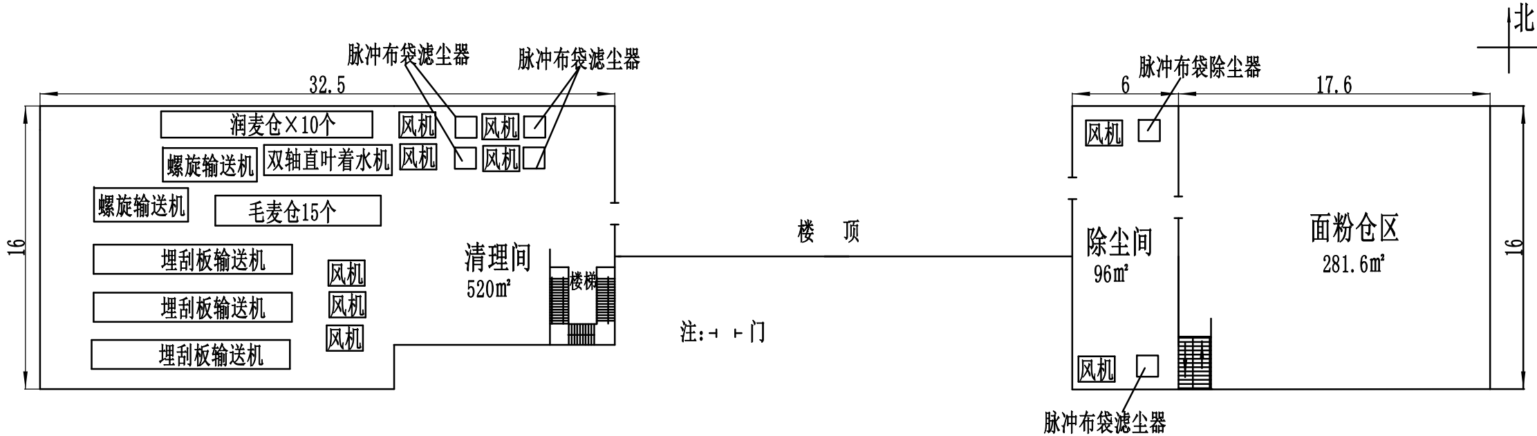
河北惠达面业有限公司生产设备布局图八（七层）
