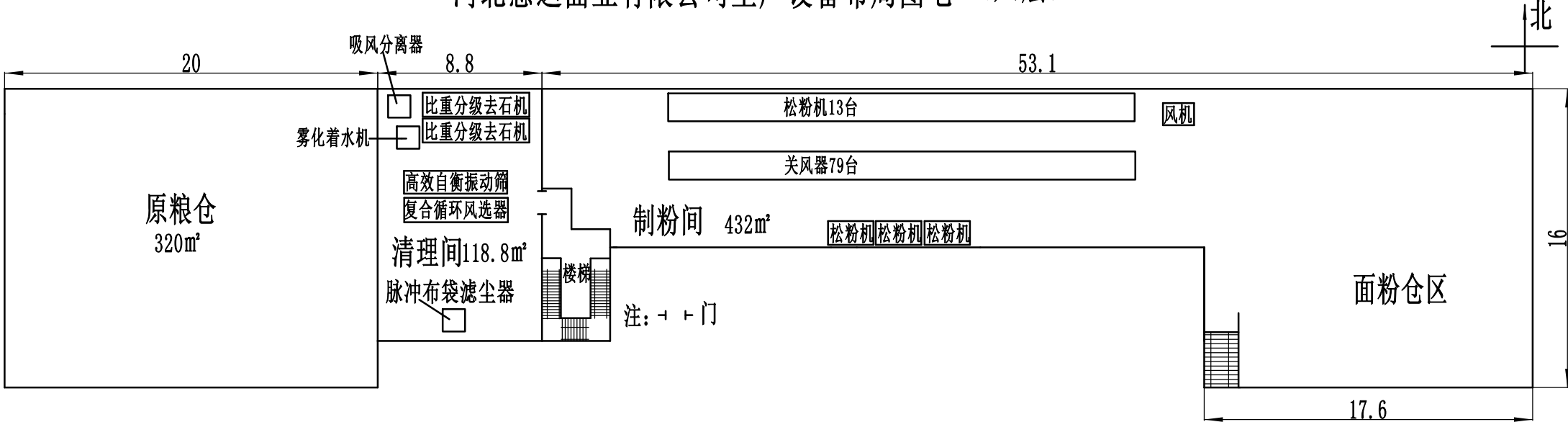
河北惠达面业有限公司生产设备布局图七（六层）
