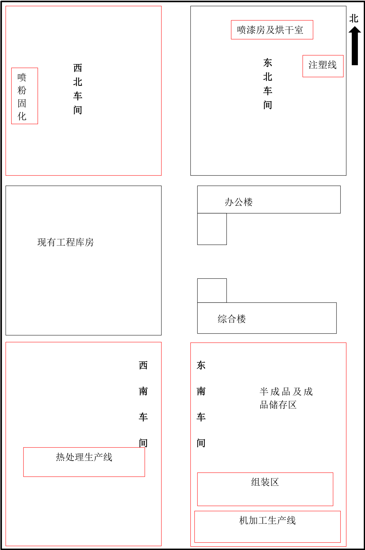
附图 3 项目所在厂区平面布置图
