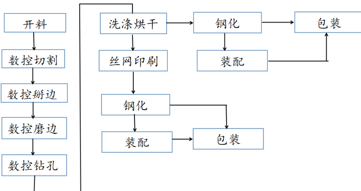
汽车钢化工艺流程图
