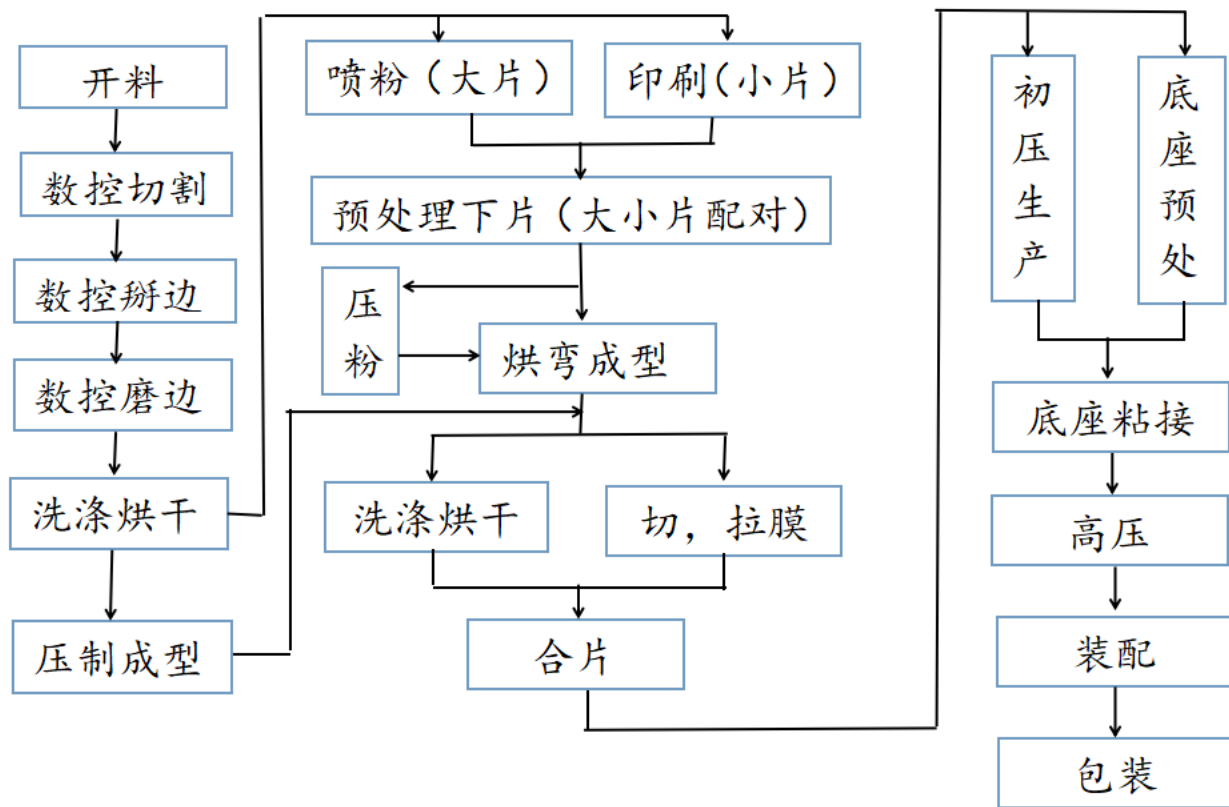
汽车夹层工艺流程图
