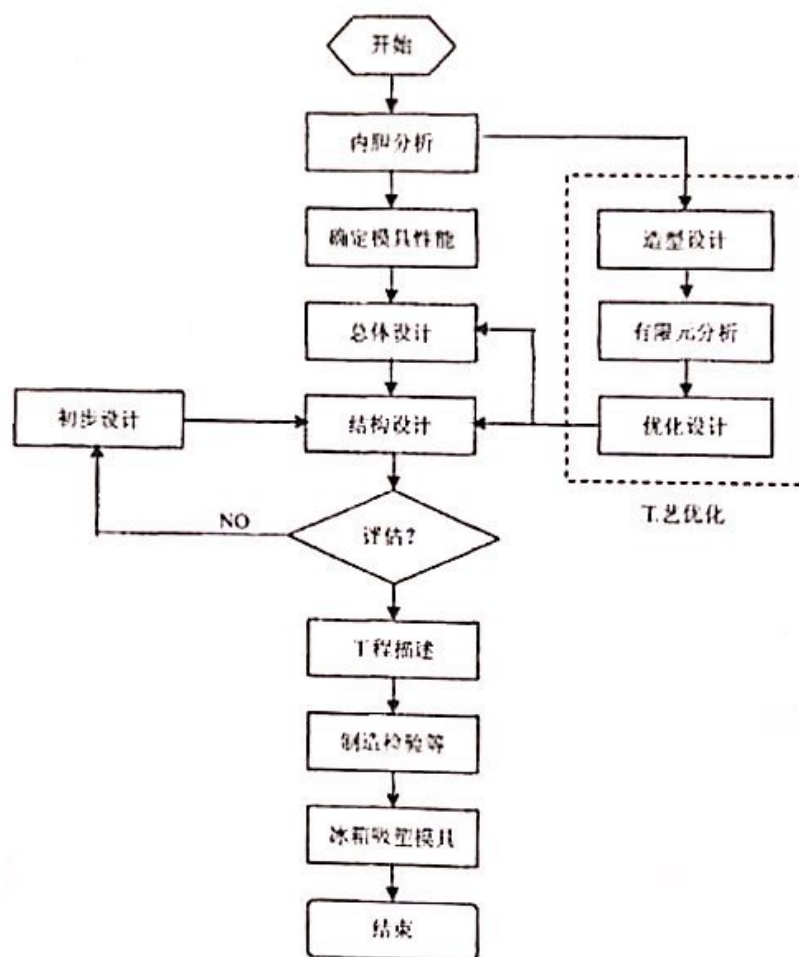
a、冰箱吸塑模具生产流程图
