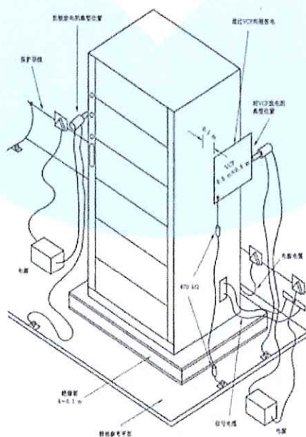
图 5 实验室试验时,落地式设备试验布置的实例
