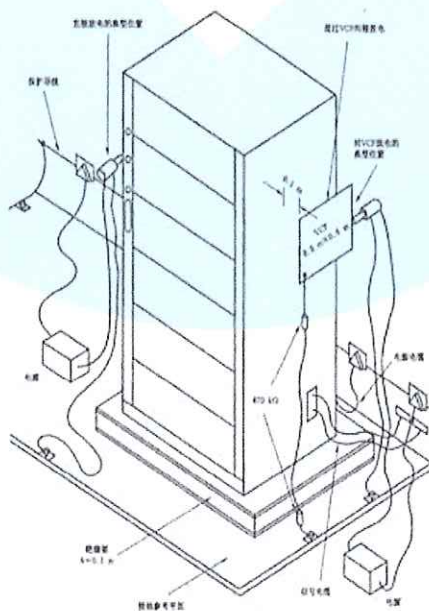
图 6 实验室试验时,落地式设备试验布置的实例
