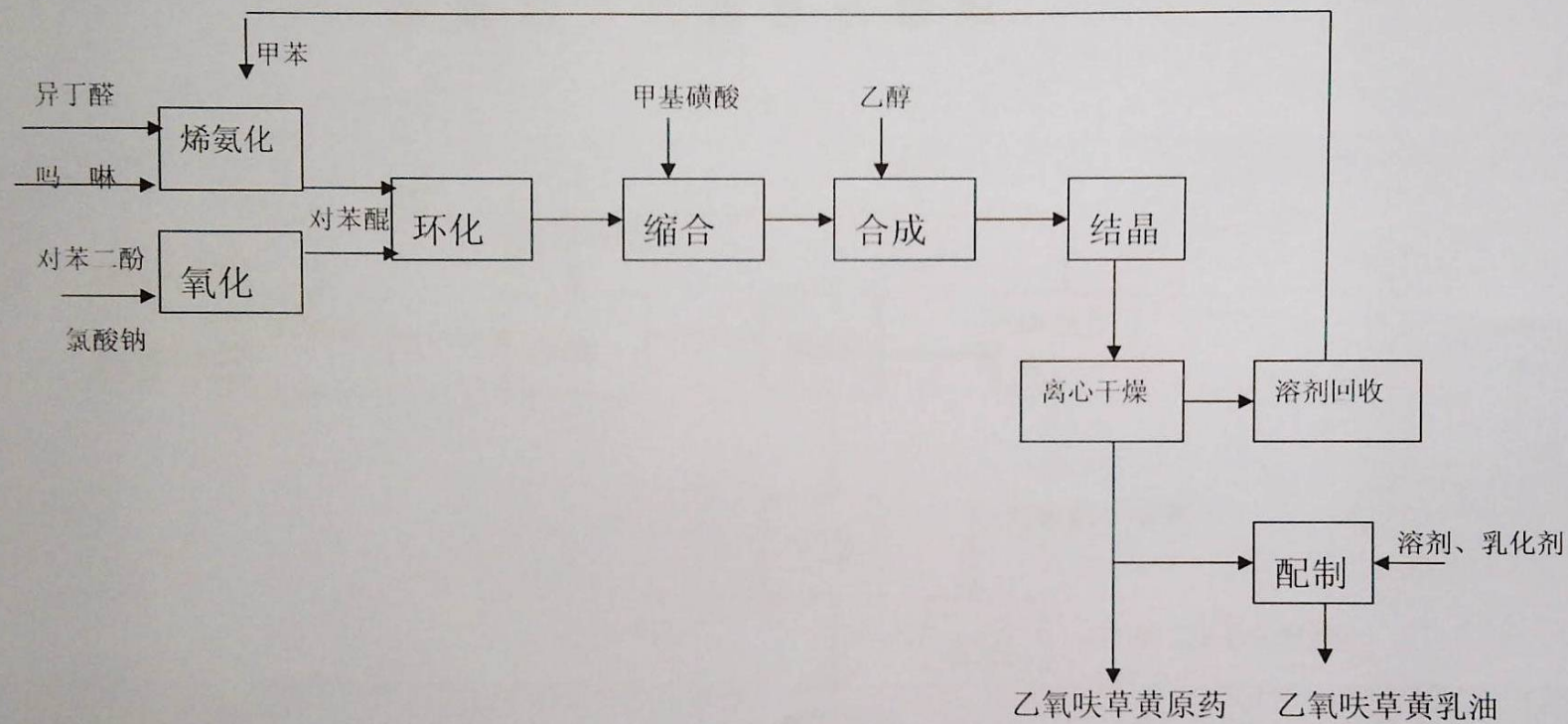
乙氧呋草黄工艺流程示意图
