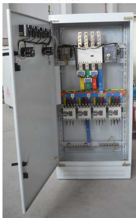
内部结构
