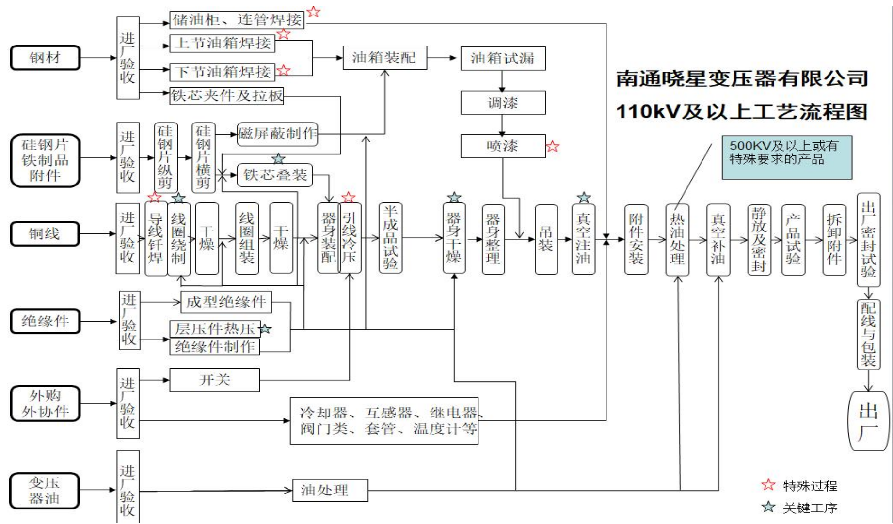
工艺流程图
